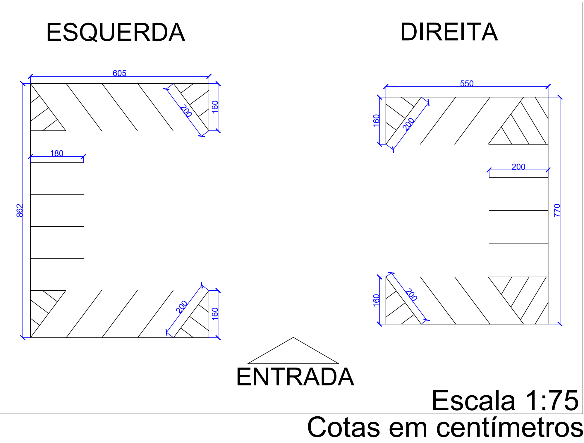
Layout para demarcação de novas vagas para carros
