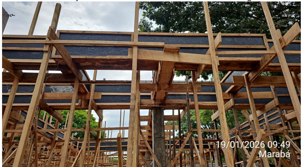
Anexo 02 – Continuação do fechamento das laterais das fôrmas das vigas:
