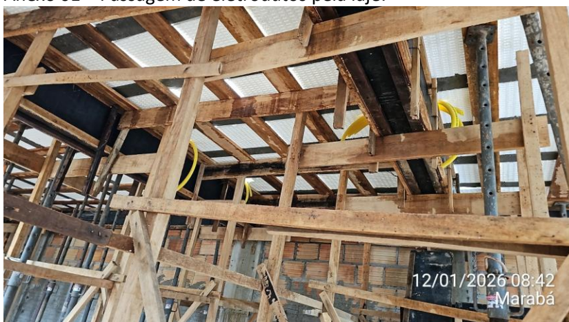
Anexo 01 – Passagem de eletrodutos pela laje:
