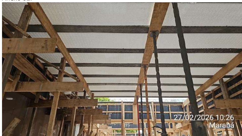
Anexo 02 – Início da colocação do escoramento metálico da laje do 2º pavimento do Anexo 02:
