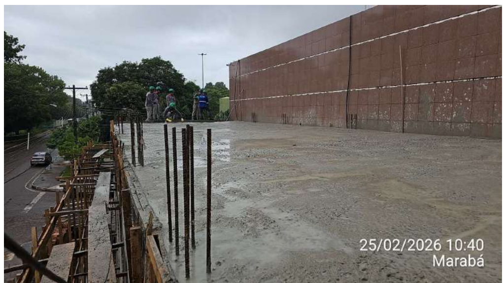
Anexo 02 – Continuação da armação das vigas da 2ª laje do Anexo 02.
