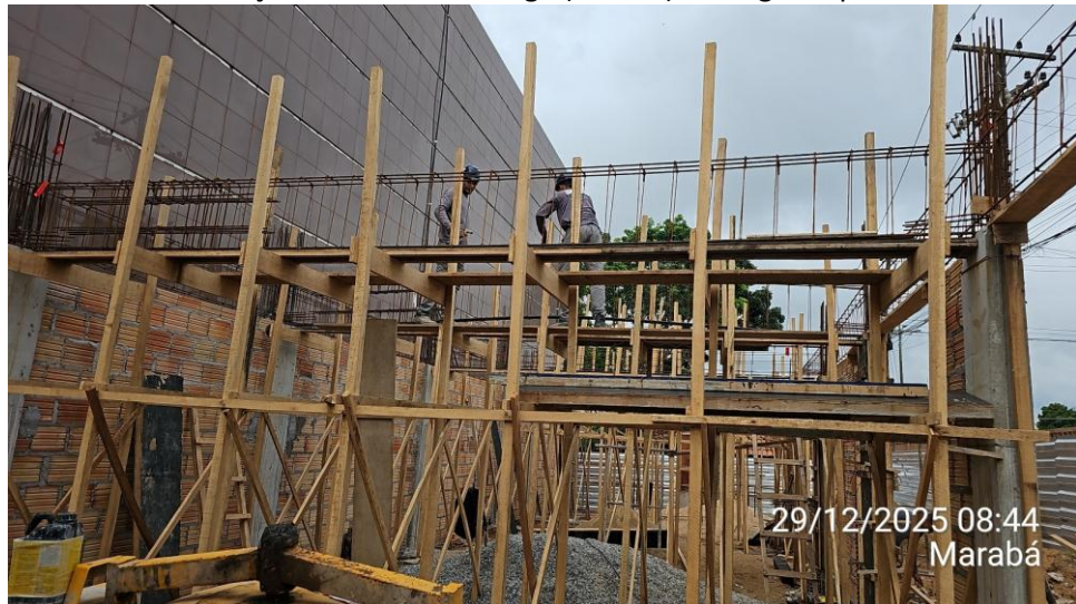
Anexo 01 – Colocação dos fundos de viga (fôrmas) das vigas superiores:
