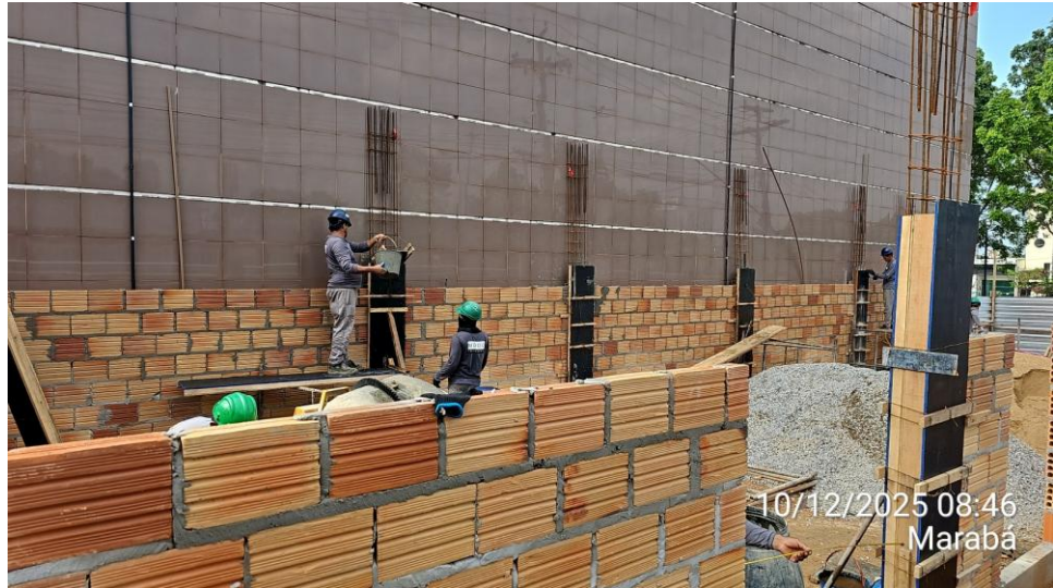
Concretagem de pilares do pavimento térreo do Anexo 01:
