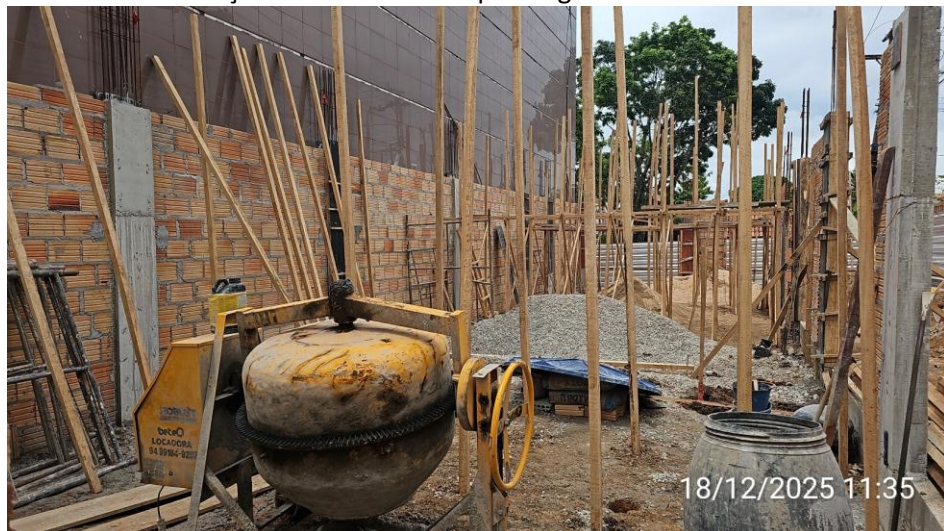
Anexo 01 – Colocação do escoramento para vigas e andaimes:
