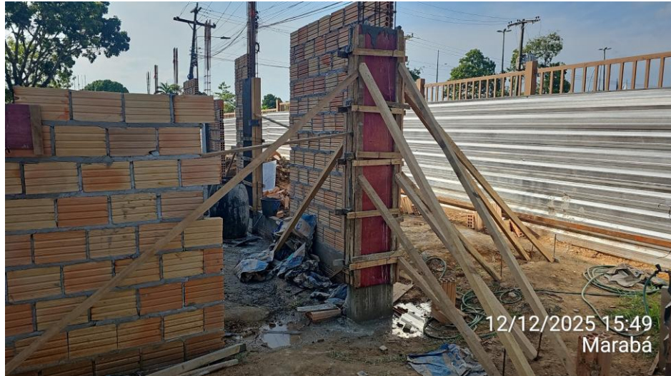
Escoramento de fôrmas de pilares do Anexo 01:
